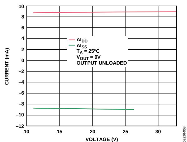
Figure 68. I_{DD}/I_{SS} vs. AV_{DD}/AV_{SS}
