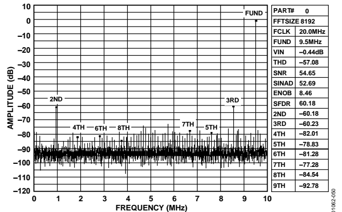
図 49. 9.5 MHz で AD9201 を AD8051 から駆動した際の FFT プロット
