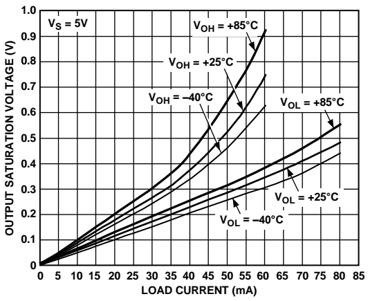
図 31. AD8051/AD8052 の負荷電流対出力飽和電圧
