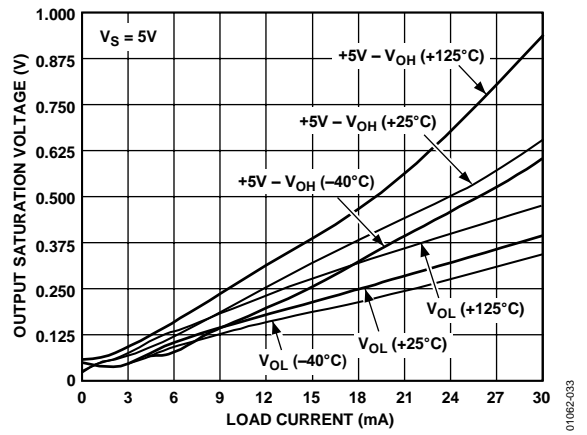
図 33. AD8054 の負荷電流対出力飽和電圧
