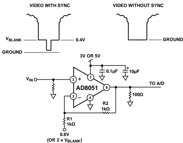
図 51.同期ストリッパ
