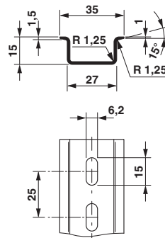
尺寸图
