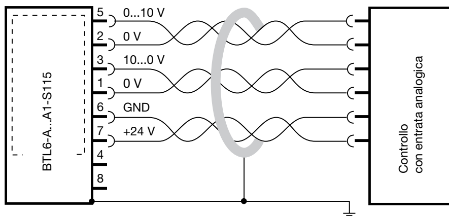
Fig. 4-1: Esempio di connessioni BTL6-A...A1-S115 con controllo
