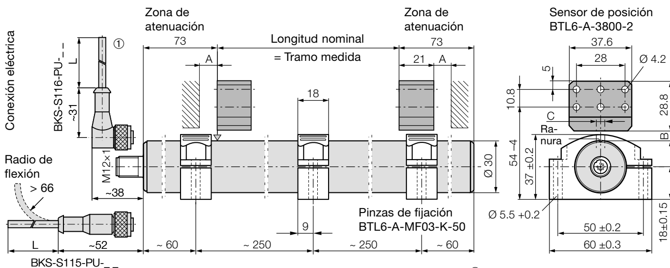
Figura 3-1: Dibujo acotado (transductor de desplazamiento BTL6...A1-S115 con sensor de posición BTL6-A-3800-2 y pinzas de fijación BTL6-A-MF03-K-50)
