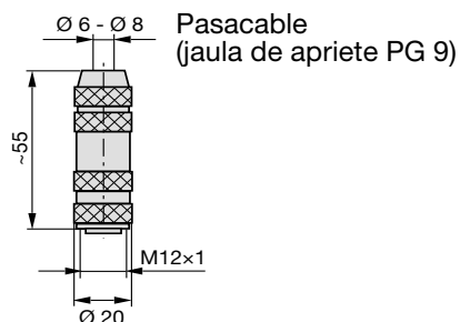
Figura 4-3: Unión de enchufe (casquillo)
