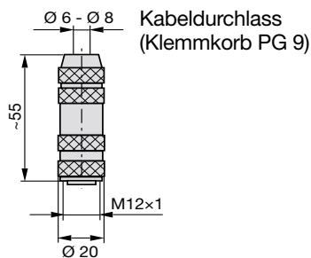
Bild 4-3: Steckverbinder (Buchse)
