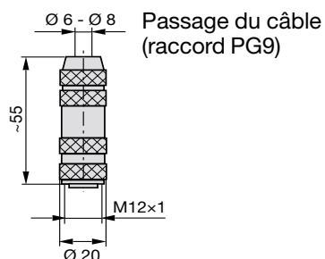
Fig. 4-3 : Connecteur (douille)
