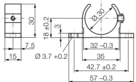
Bild 7-2: Befestigungsklammer BTL6-A-MF01-A-43
