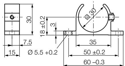
Bild 7-1: Befestigungsklammer BTL6-A-MF01-A-50
