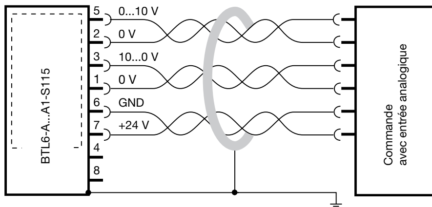
Fig. 4-1 : Exemple de raccordement BTL6-A...A1-S115 avec commande
