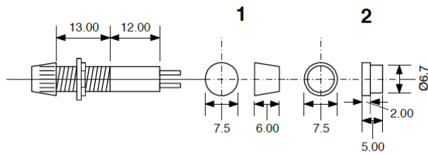
Body Dimensions
