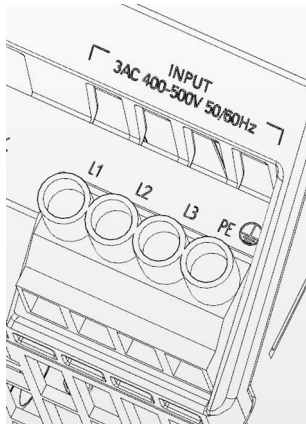
Bild 3: Input ① Figure 3: Input ① Figure 3: Input ① Figura 3: Entrada ①
