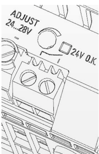
Bild 7: Meldekontakt ③ Figure 7: Signaling contact ③ Figure 7: Contact de signalisation ③ Figura 7: Contatto di segnalazione ③ Figura 7: Contacto de señalización ③
