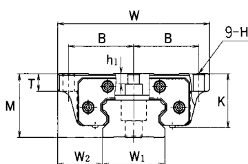
HSR-HB Type
