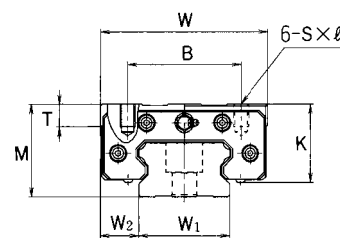
HSR-HR Type
