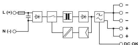
结构框图
