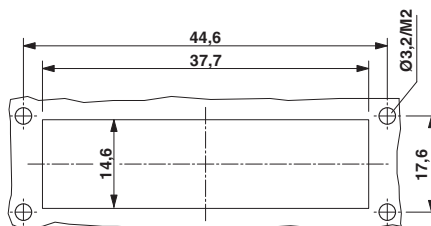
尺寸图
