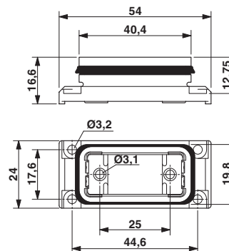
尺寸图
