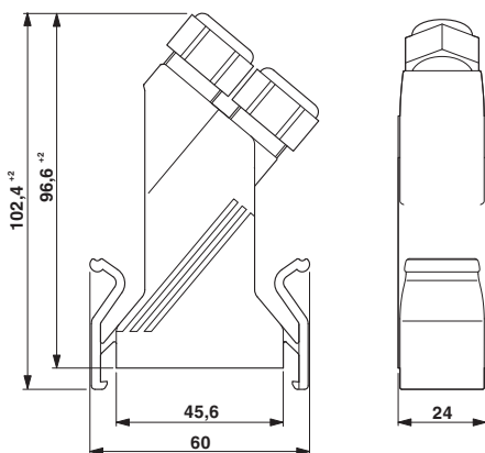
尺寸图
