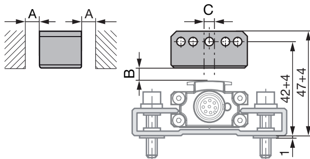
Fig. 4-6 : Dimensions et distances pour le capteur de position BTL6-A-3801-2
