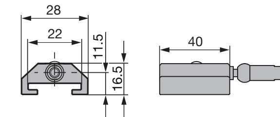
Fig. 11-6: Dimensioni di ingombro datore di posizione BTL5-T-2814-1S
