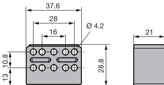
Bild 11-3: Einbaumaße Positionsgeber BTL6-A-3800-2
