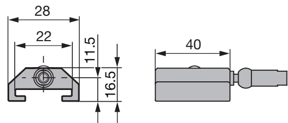
Bild 11-6: Einbaumaße Positionsgeber BTL5-T-2814-1S
