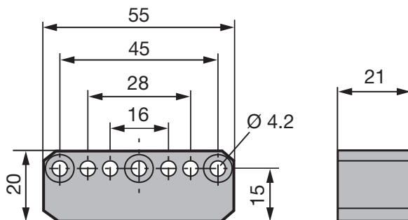
Bild 11-2: Einbaumaße Positionsgeber BTL5-P-5500-2
