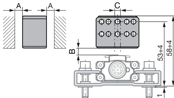
Fig. 4-5: Medidas y distancias con el sensor de posición BTL6-A-3800-2
