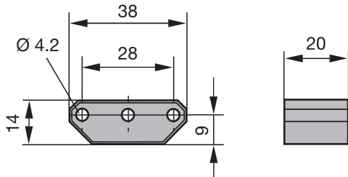
Fig. 11-1 : Dimensions de montage du capteur de position BTL5-P-3800-2
