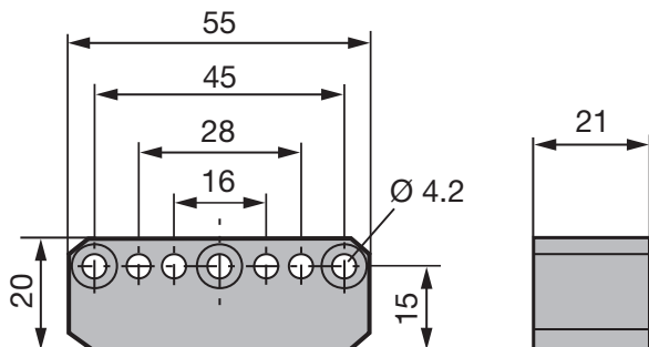
Fig. 11-2 : Dimensions de montage du capteur de position BTL5-P-5500-2
