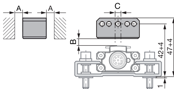
Fig. 4-6: Medidas y distancias con el sensor de posición BTL6-A-3801-2
