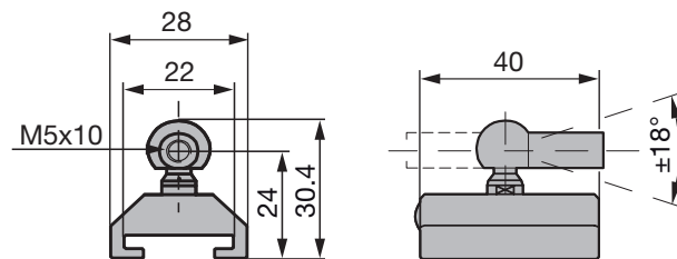
Fig. 11-5 : Dimensions de montage du capteur de position BTL5-F-2814-1S
