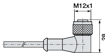
Bild 11-10: Conector BKS-S116-PU- _ _
