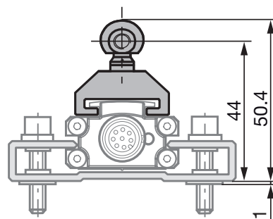
Fig. 4-1: Medidas y distancias con el sensor de posición BTL5-F-2814-1S
