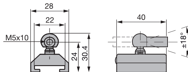
Fig. 11-5: Dimensioni di ingombro datore di posizione BTL5-F-2814-1S
