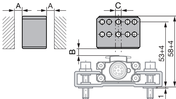
Fig. 4-5 : Dimensions et distances avec le capteur de position BTL6-A-3800-2
