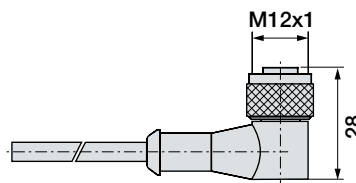
Bild 11-10: Steckverbinder BKS-S116-PU- _ _
