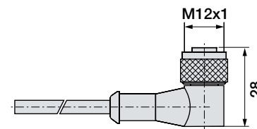
Bild 11-10: Connettore BKS-S116-PU- _ _
