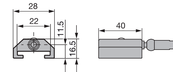
Fig. 11-6 : Dimensions de montage du capteur de position BTL5-T-2814-1S
