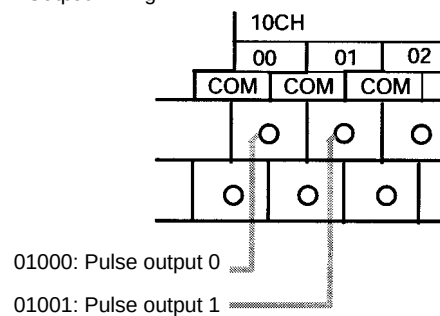
Output Wiring
