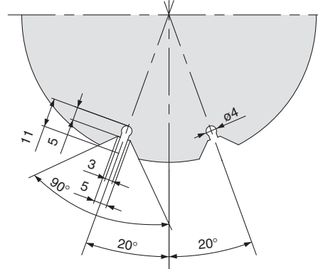
MHSJ3-80D
