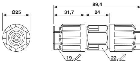
尺寸图
