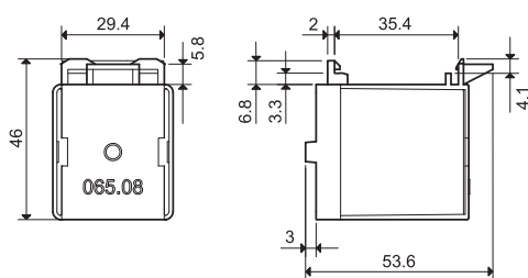
Rear 35 mm rail (EN 60715) mount for types 65.31.xxxx.xxx9
