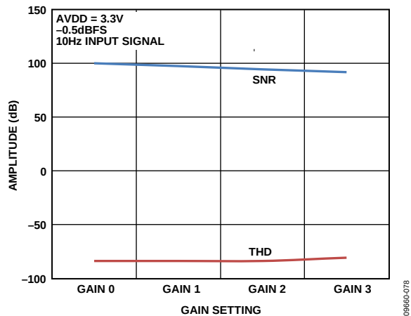
图49. 不同增益设置下的SNR和THD
