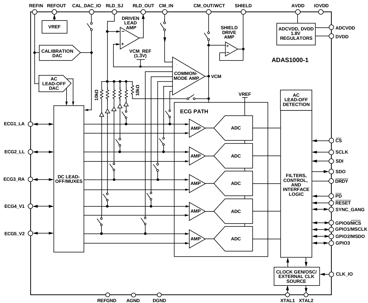
图54. ADAS1000-1简化功能框图
