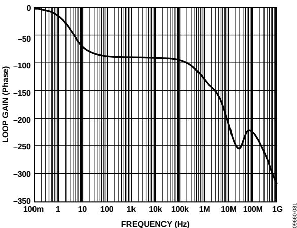
图52. 无负载时 ADAS1000 右腿驱动放大器的开环相位响应
