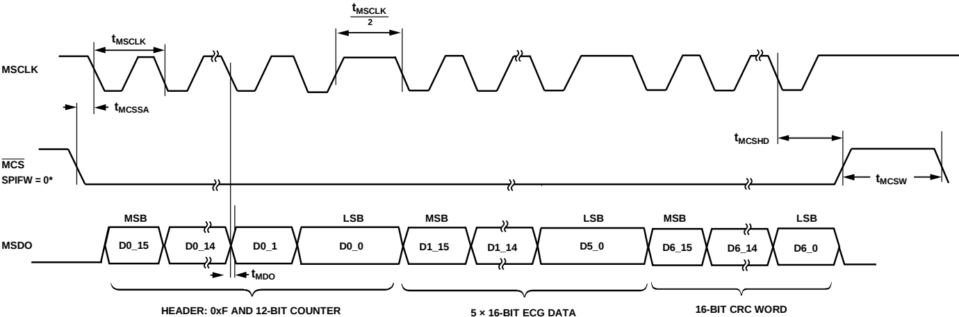
图5. SPIFW = 0时的数据读取和写入时序图, 显示整个包的数据(表头、5个ECG字和CRC字)
