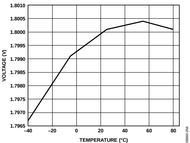
图29. 典型内部VREF与温度的关系
