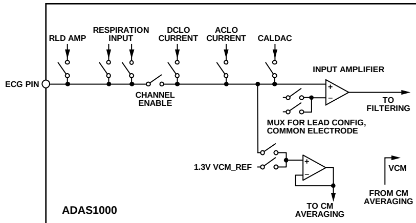
图63. 典型ECG通道输入复用
