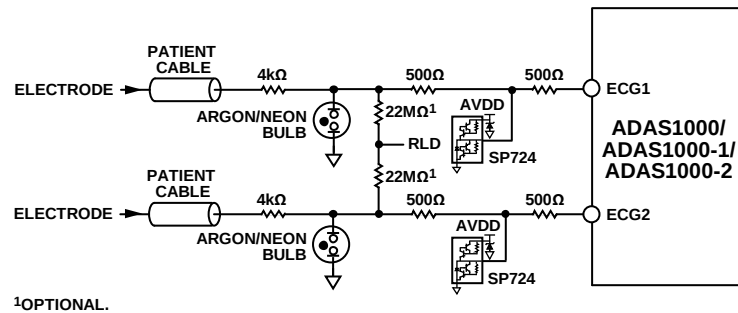
图61. ECG路径上的除颤保护示例——使用氖泡
