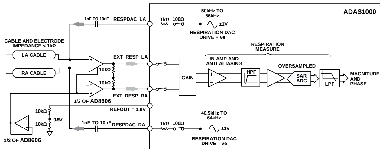
图68. 使用外部电容和外部放大器的呼吸测量
