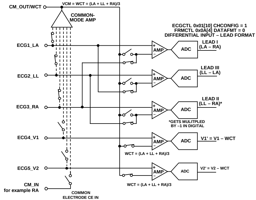
图58. 灵活的前端配置—相对于威尔逊中心电端(WCT)的模拟导联模式配置
