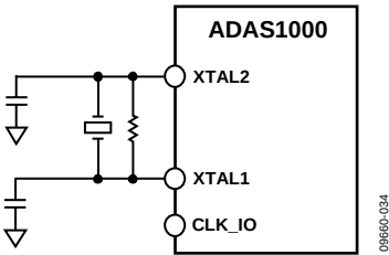
图77. 输入时钟
