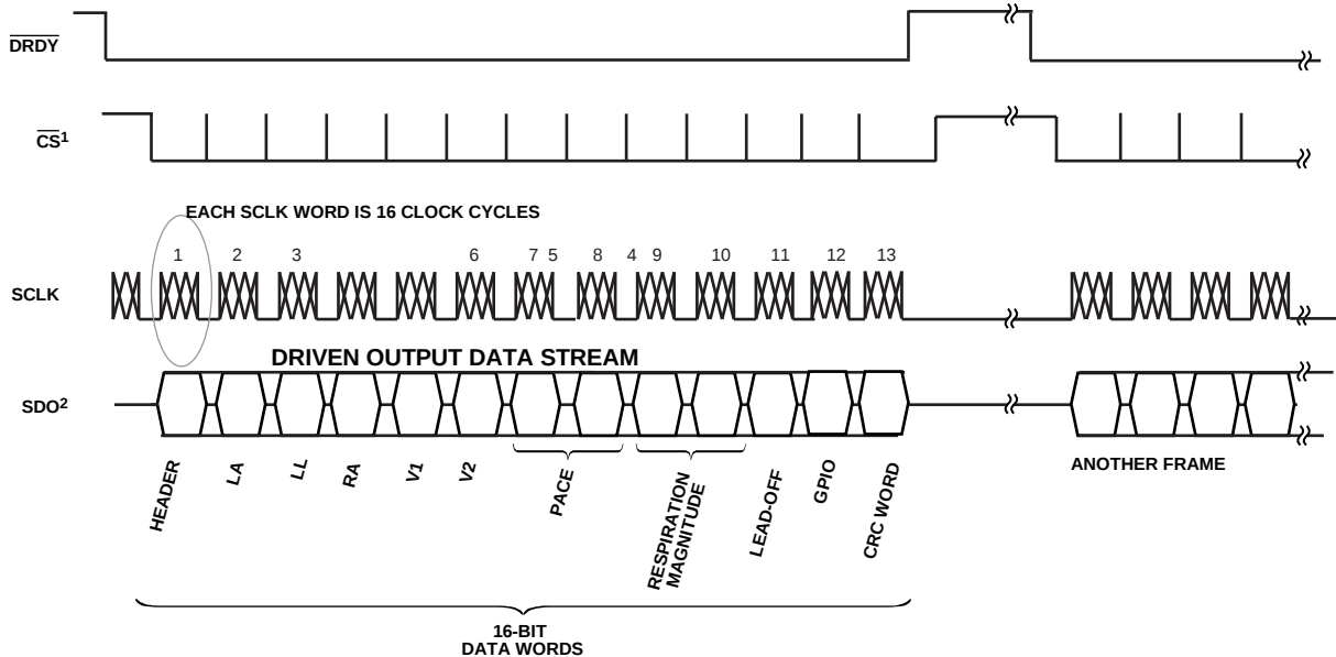
图79. 2 kHz和16 kHz数据速率的输出帧结构，SDO数据配置为电极或导联数据
