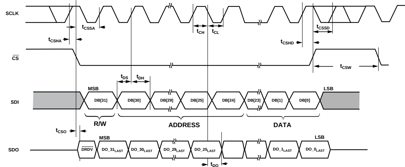
图2. 数据读取和写入时序图(CPHA = 1、CPOL = 1)
