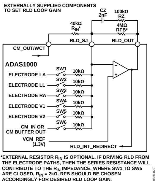
图65. 右腿驱动——可能的外部器件配置
