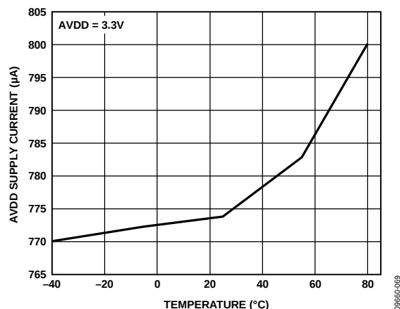
图33. 典型AVDD电源电流与温度的关系，待机模式
