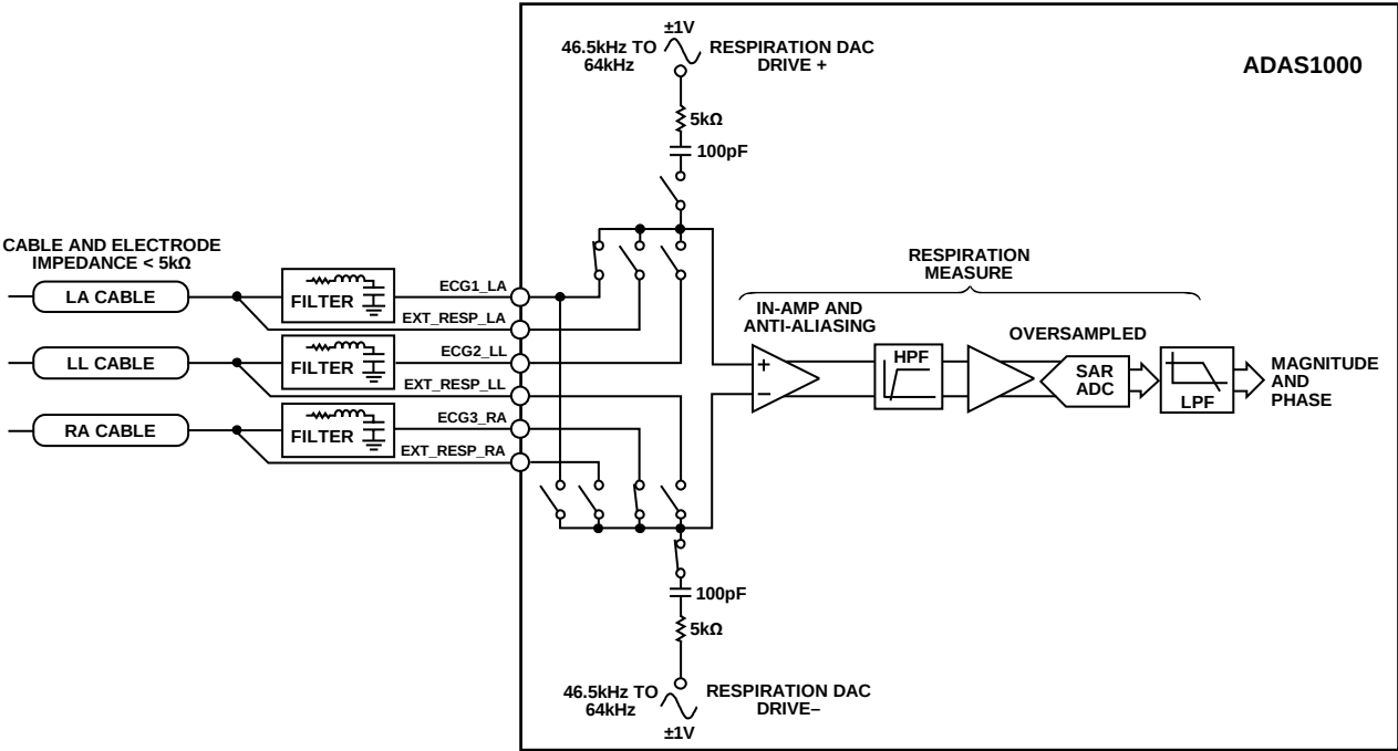
图66. 呼吸简化功能框图
