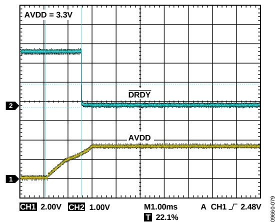
图50. AVDD线上电至DRDY变为低电平(就绪)
