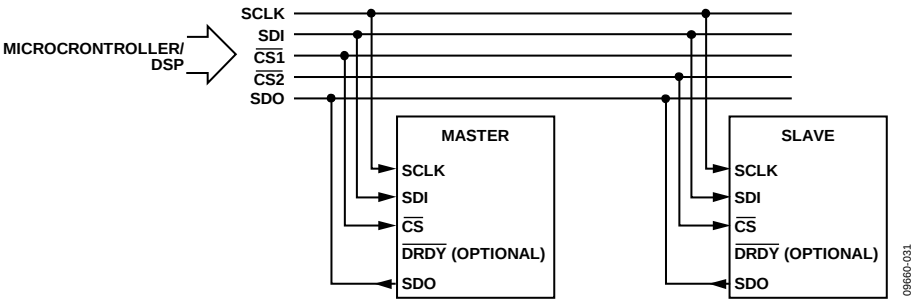
图75. 多个器件接口的一种方法
