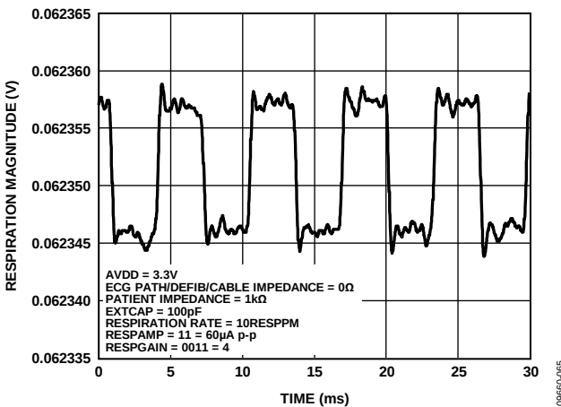
图38. 200 mΩ阻抗变化下的呼吸，使用外部呼吸DAC驱动100 pF外部电容，利用0 Ω病人电缆测量
