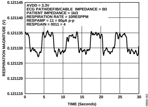
图36. 100 mΩ阻抗变化下的呼吸，使用内部呼吸路径，利用0 Ω病人电缆测量
