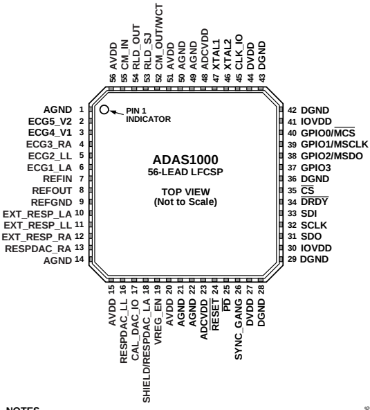
图8. ADAS1000 56引脚LFCSP引脚配置
