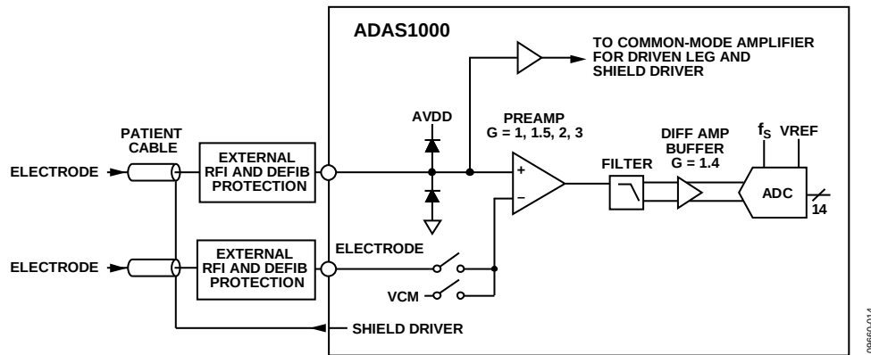
图56. 单个ECG通道的简化示意图
