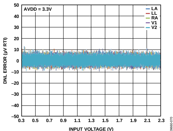
图42. 不同电极、25°C时的DNL与输入电压范围的关系
