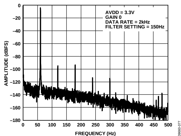
图48. 60 Hz输入信号下的FFT
