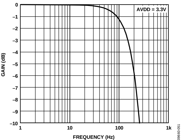
图24. 滤波器响应：150 Hz滤波器使能、2 kHz数据速率； 数字滤波器概况见图72
