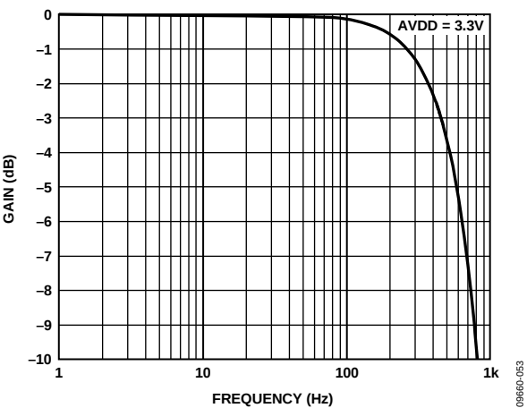
图26. 滤波器响应：450 Hz滤波器使能、2 kHz数据速率； 数字滤波器概况见图72
