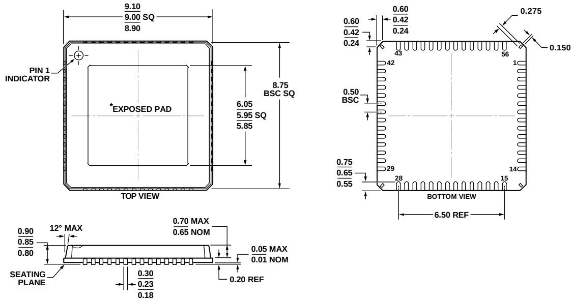
图82. 56引脚引脚架构芯片级封装[LFCSP_VQ]
