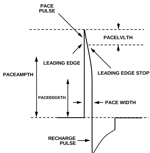
图71. 典型起搏信号
