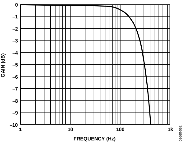
图25. 滤波器响应：250 Hz滤波器使能、2 kHz数据速率； 数字滤波器概况见图72
