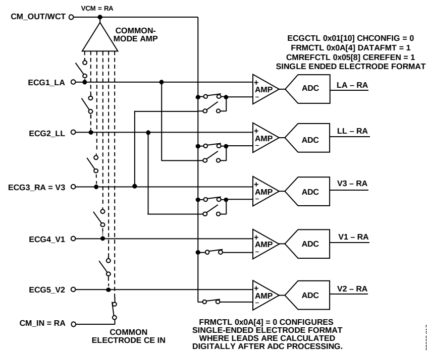
图60. 灵活的前端配置—公共电极配置
