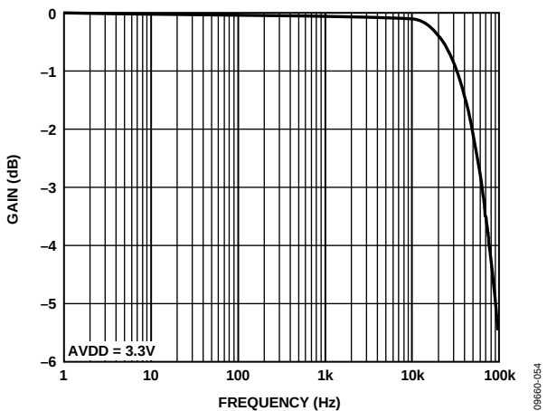
图27. 模拟通道带宽
