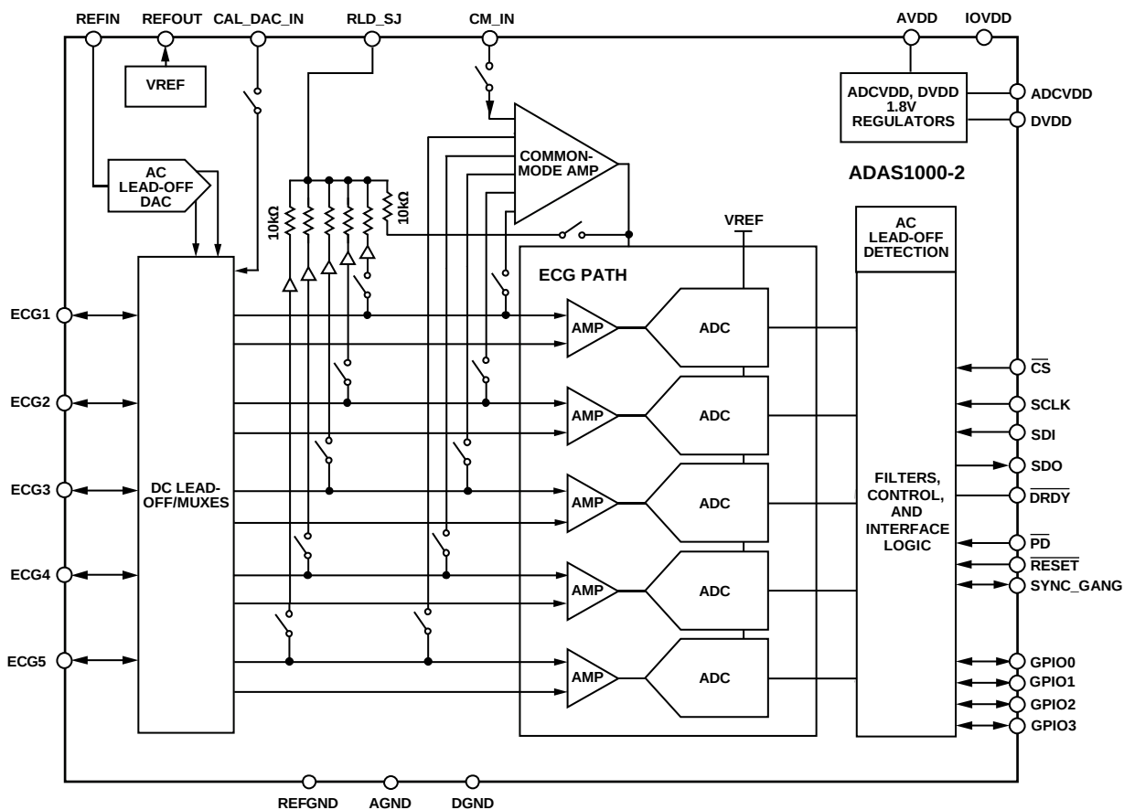
图55. ADAS1000-2从器件简化功能框图
