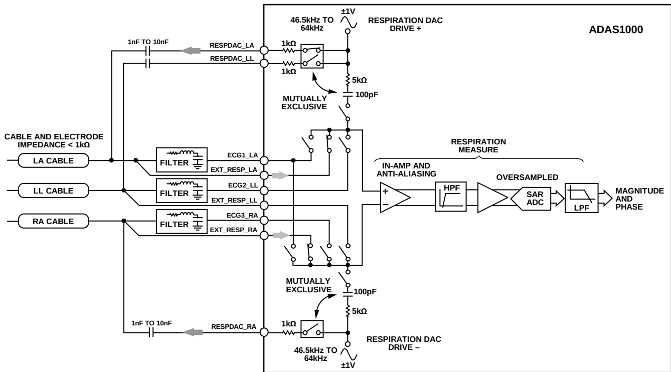
图67. 使用外部电容的呼吸测量
