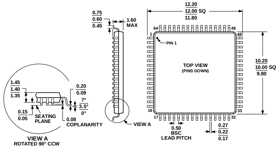
图83. 64引脚薄型四方扁平封装[LQFP]
