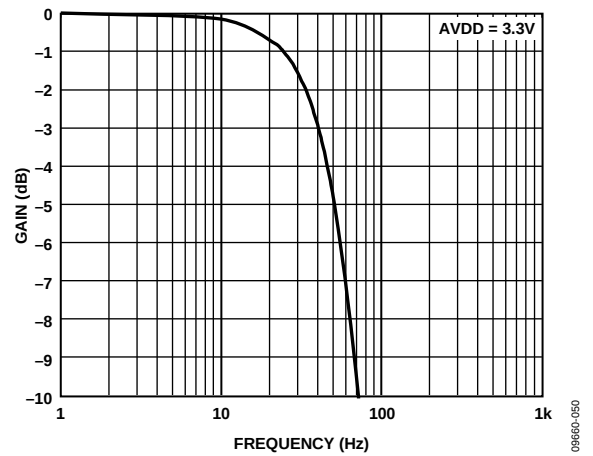
图23. 滤波器响应: 40 Hz滤波器使能、2 kHz数据速率; 数字滤波器概况见图72
