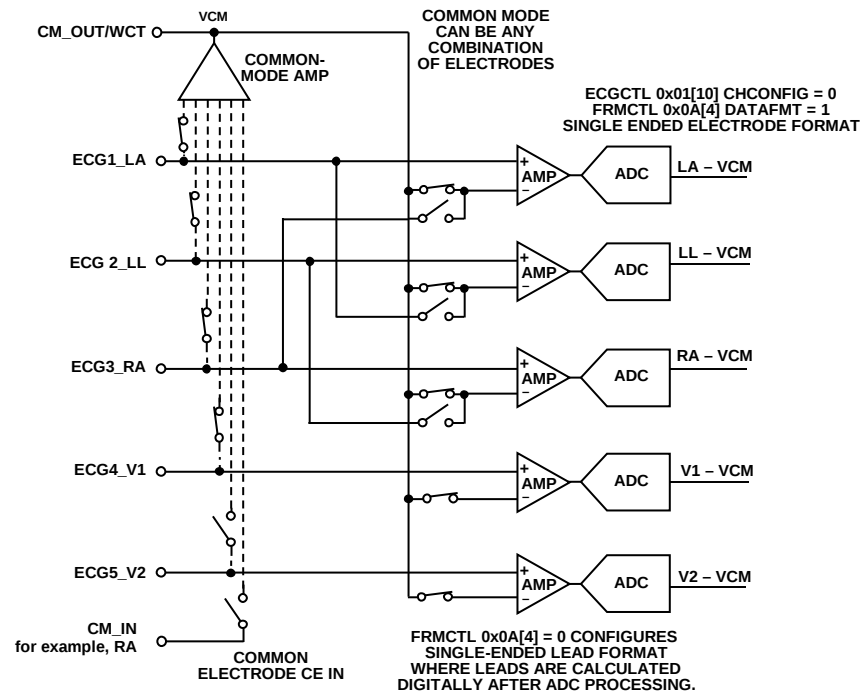
图59. 灵活的前端配置—单端电极配置
