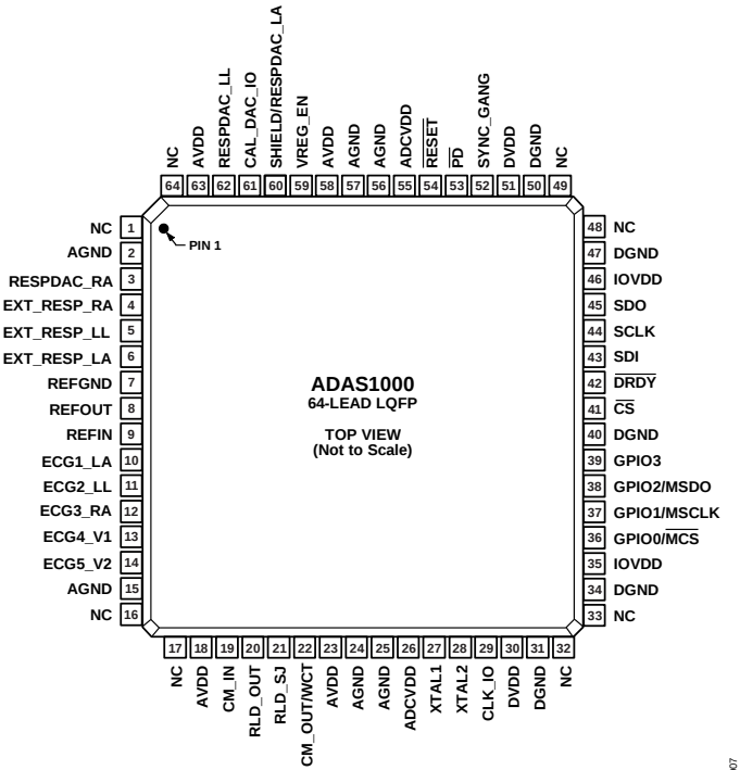
图7. ADAS1000 64引脚LQFP引脚配置
