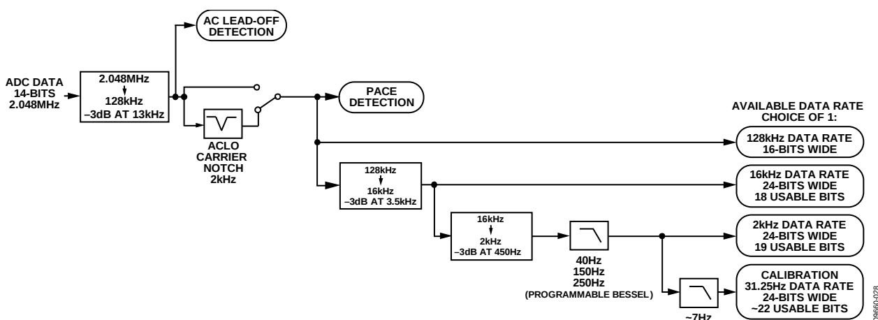
图72. ECG通道滤波器信号流
