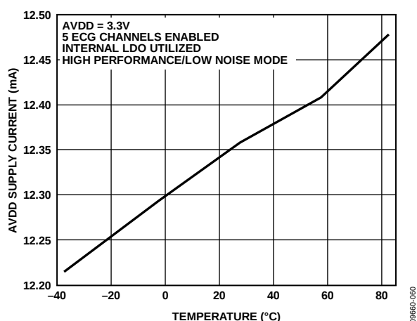
图31. 典型AVDD电源电流与温度的关系，使用内部ADVCDD/DVDD电源
