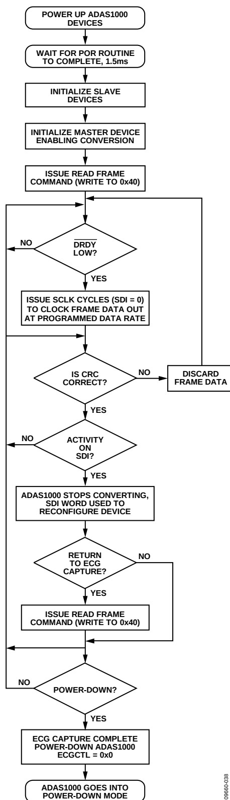
图81. 与多个ADAS1000/ADAS1000-1/ADAS1000-2器件接口的建议软件流程图
