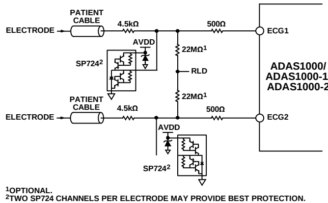
图62. ECG路径上的除颤保护示例——使用二极管保护
