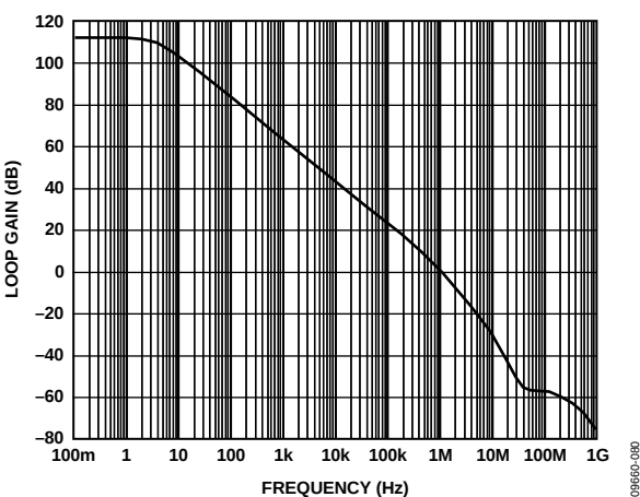
图51. 无负载时 ADAS1000 右腿驱动放大器的开环增益响应
