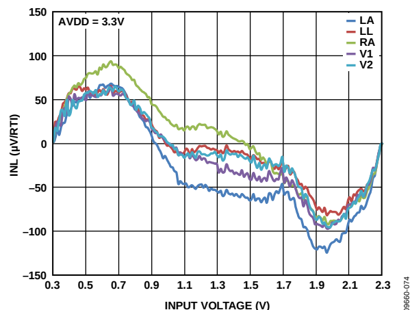
图45. 不同电极通道的INL与输入电压的关系，2 kHz数据速率
