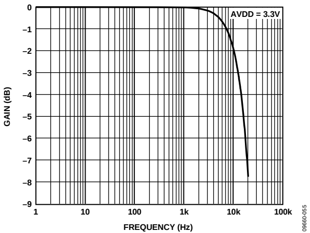
图28. 滤波器响应：128 kHz数据速率； 数字滤波器概况见图72
