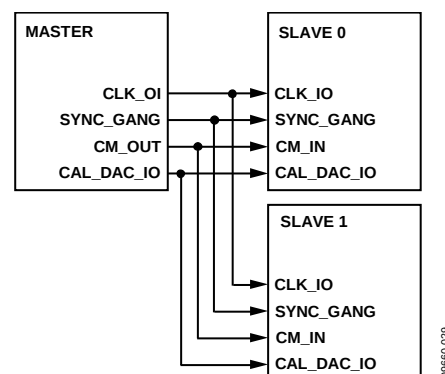
图73. 组合模式下的主/从连接，使用多个ADAS1000/ADAS1000-1/ADAS1000-2器件
