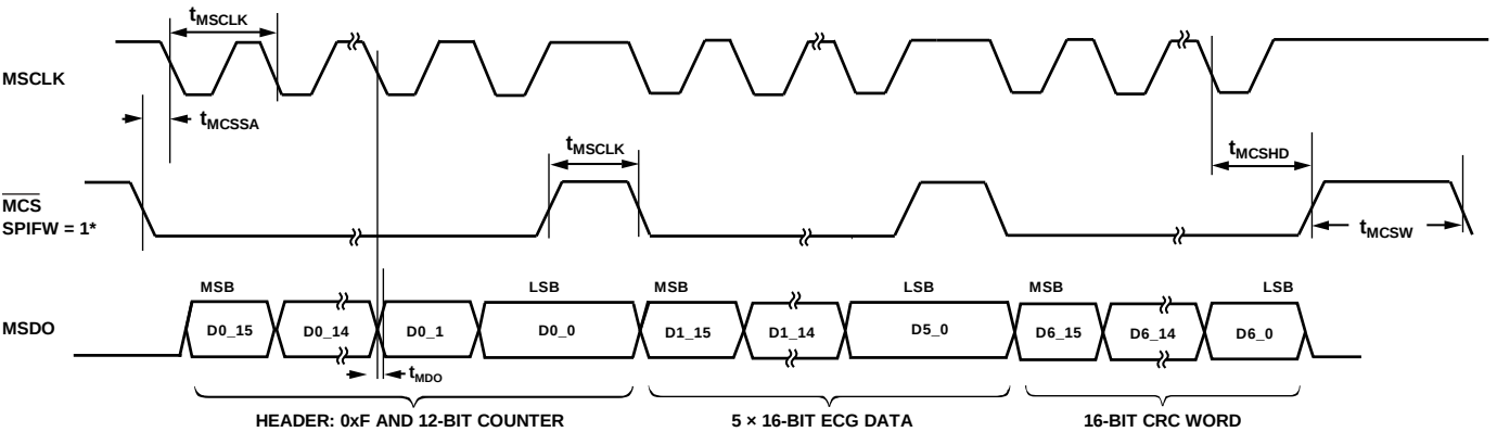
图6. SPIFW = 1时的数据读取和写入时序图, 显示整个包的数据(表头、5个ECG字和CRC字)
