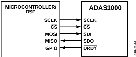
图76. 串行接口
