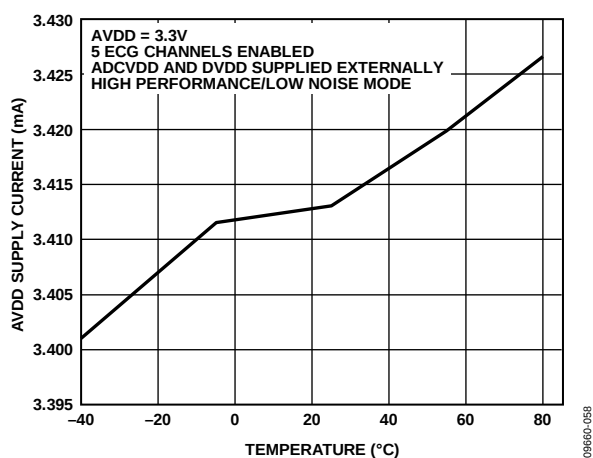
图32. 典型AVDD电源电流与温度的关系，使用外部提供的ADVCDD/DVDD
