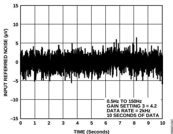
图15. 折合到输入端噪声: 0.5 Hz至150 Hz带宽, 2 kHz数据速率, GAIN 3 (4.2)
