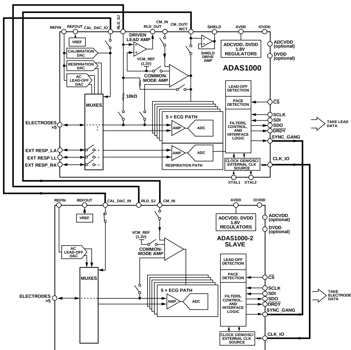
图74. 配置多个器件以扩大电极/导联数量 (此例将ADAS1000用作主器件，ADAS1000-2用作从器件。类似地，ADAS1000-1也可以用作主器件)
