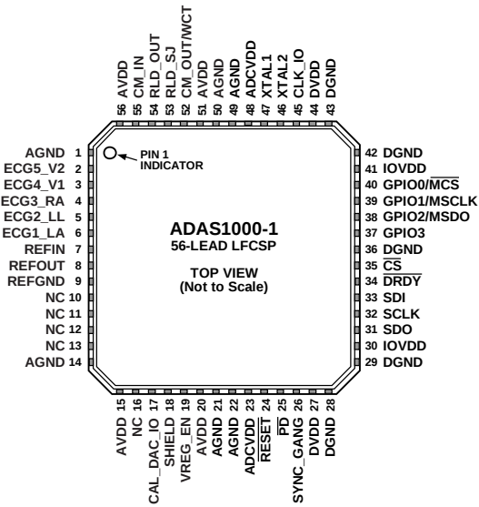
图9. ADAS1000-1 56引脚LFCSP引脚配置
