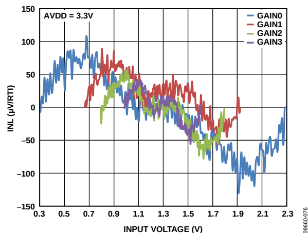
图47. 不同增益设置下的INL与输入电压的关系，128 kHz数据速率
