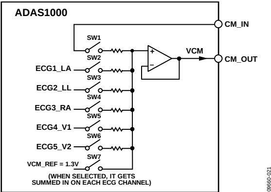
图64. 共模产生模块
