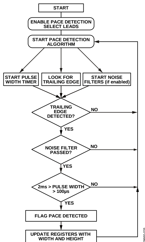
图70. 起搏算法概览
