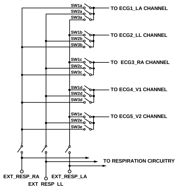
图69.呼吸路径的其它用途
