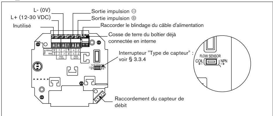
Fig. 3.6 Connexion SE35, 12-30 VDC, sans relais, avec presse-étoupes
