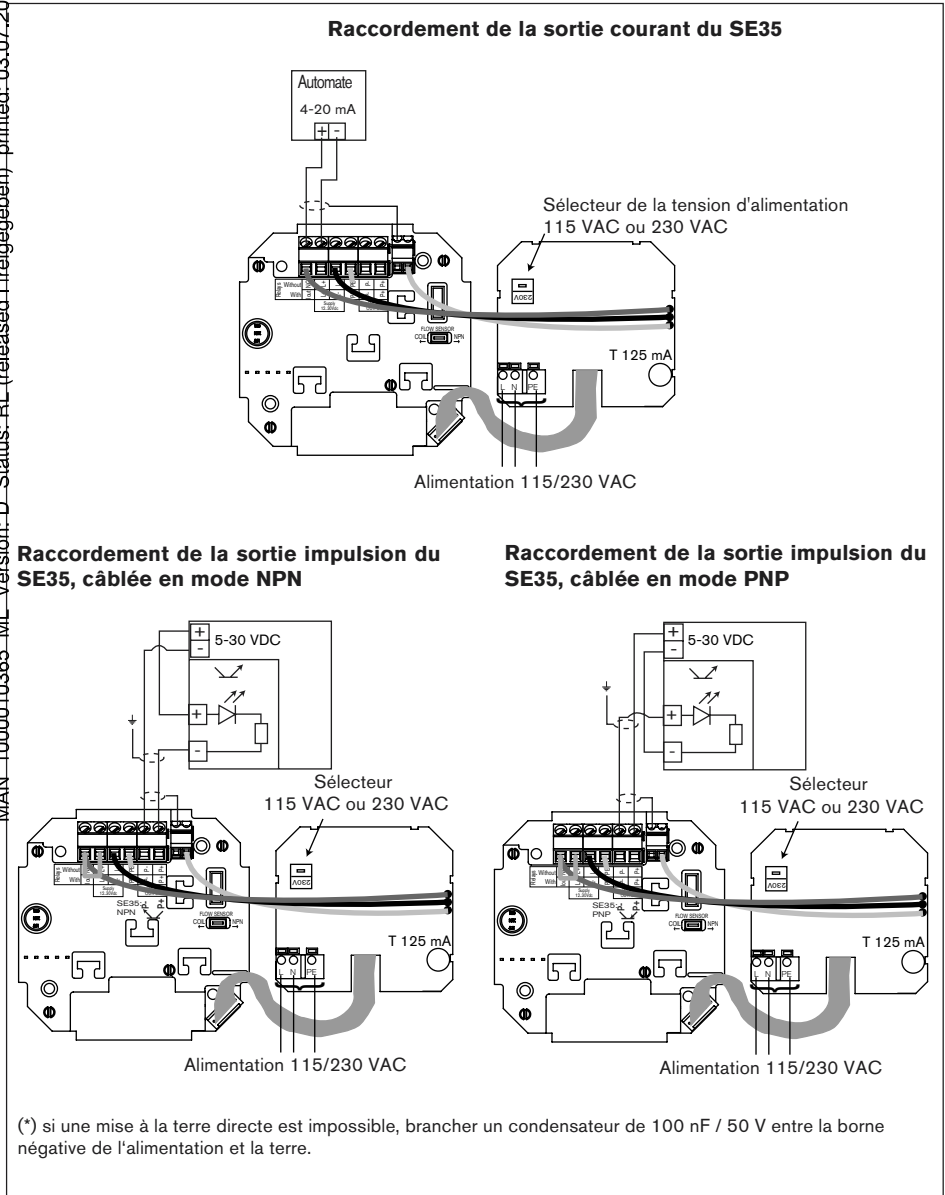
Fig. 3.11 Raccordement du module électronique SE35, 115/230 VAC, sans relais, avec presse-étoupe, à un automate
