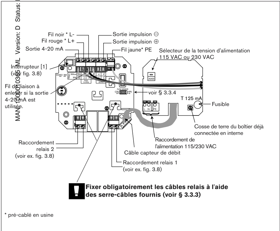
Fig. 3.12 Connexion SE35, 115/230 VAC, avec relais et presse-étoupes
