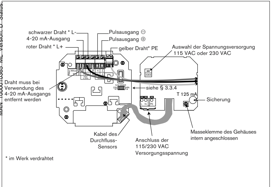
Fig. 3.10 Anschluss des SE35, 115/230 VAC, ohne Relais, mit Kabelverschraubungen
