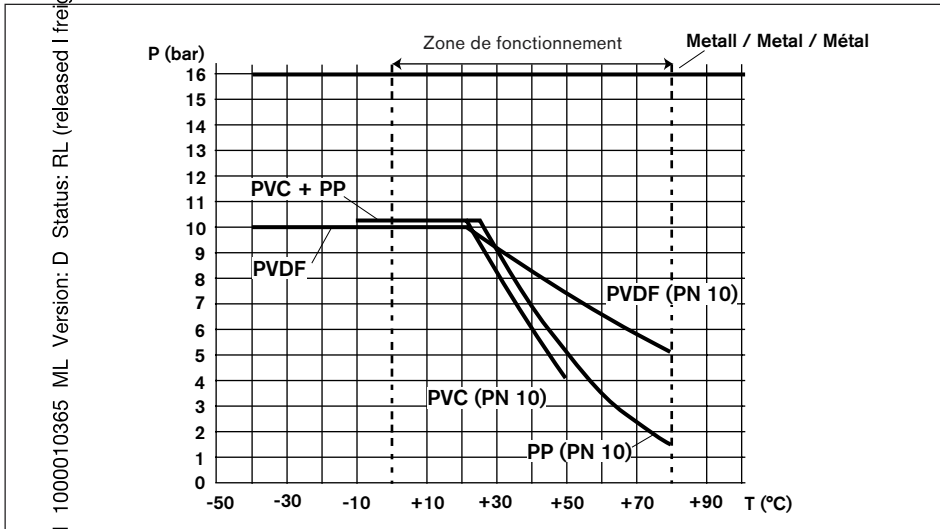
Fig. 3.1 Dépendance température-pression
