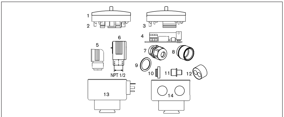
Fig. 5.1 Ersatzteil-Explosionszeichnung SE35
