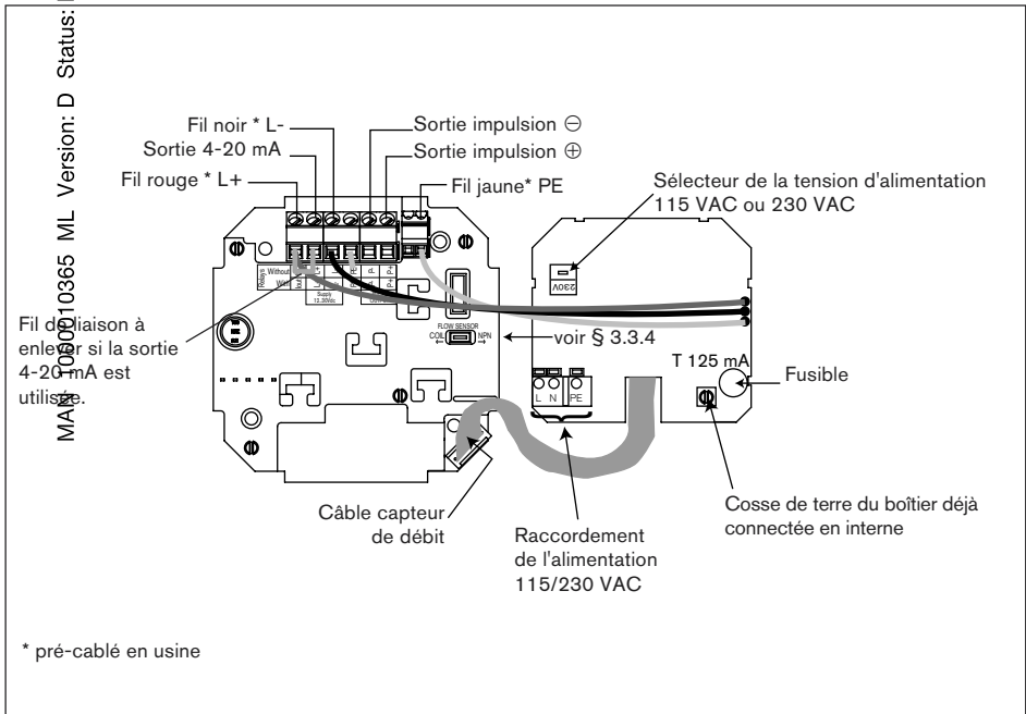
Fig. 3.10 Connexion SE35, 115/230 VAC, sans relais, avec presse-étoupes
