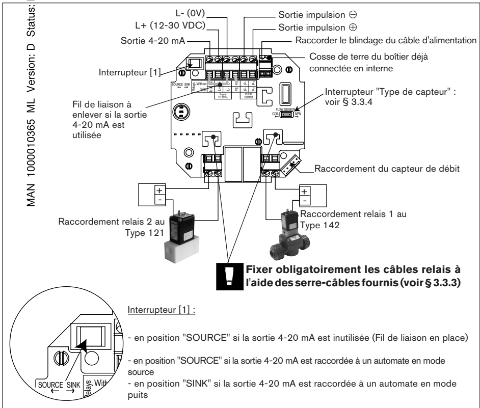
Fig. 3.8 Connexion SE35, 12-30 VDC, avec relais et presse-étoupes
