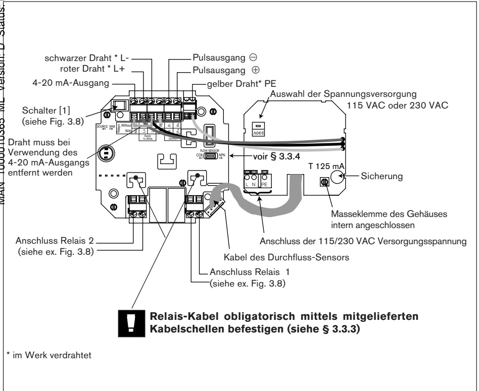
Fig. 3.12 Anschluss des SE35, 115/230 VAC, mit Relais und Kabelverschraubungen
