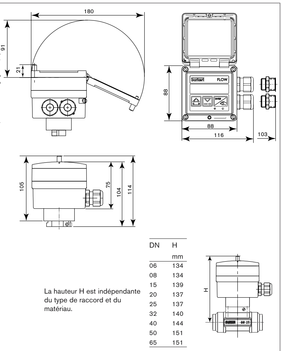
Fig. 2.1 Dimensions transmetteur de débit
