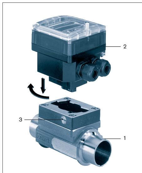
Fig. 3.2 Montage 8035
