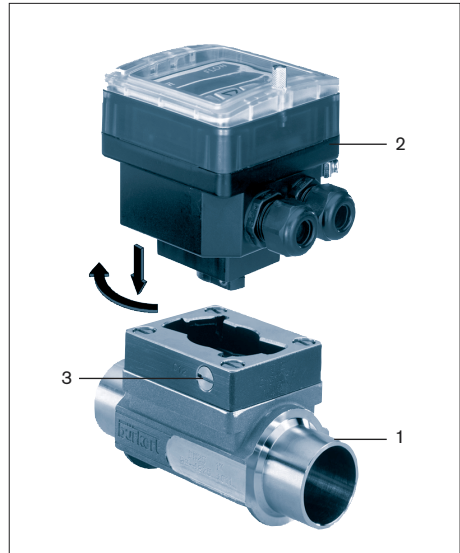
Fig. 3.2 Einbau 8035
