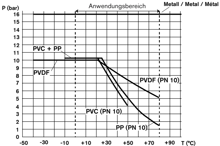
Fig. 3.1 Druck-Temperatur-diagramm
