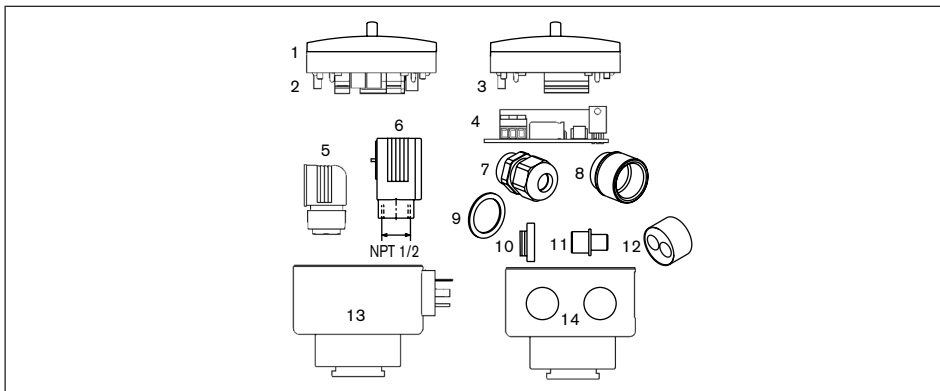
Fig. 5.1 Vue éclatée des pièces de rechange SE35
