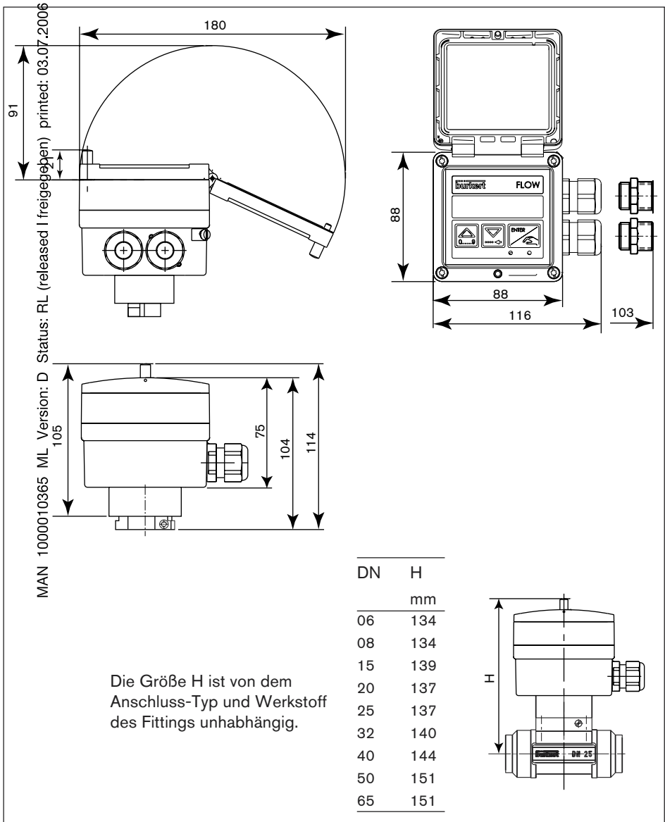
Fig. 2.1 Durchfluss-Transmitter Abmessungen
