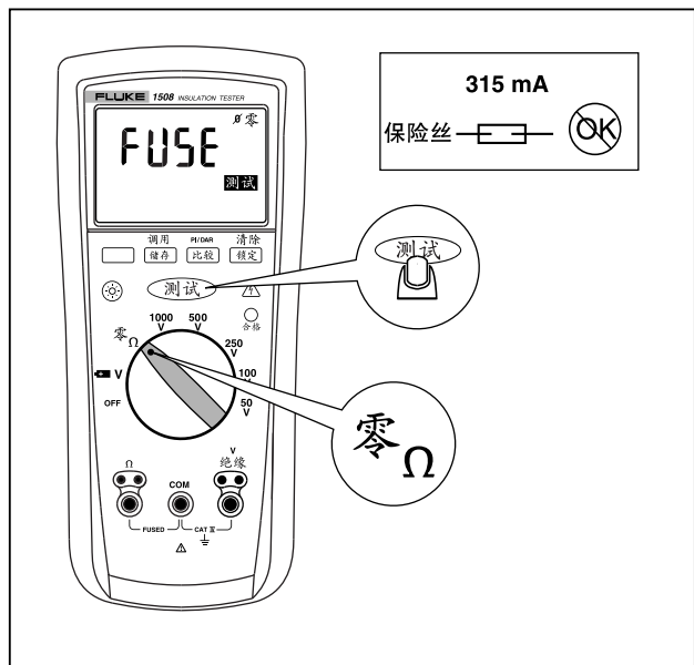
图 10. 测试保险丝
