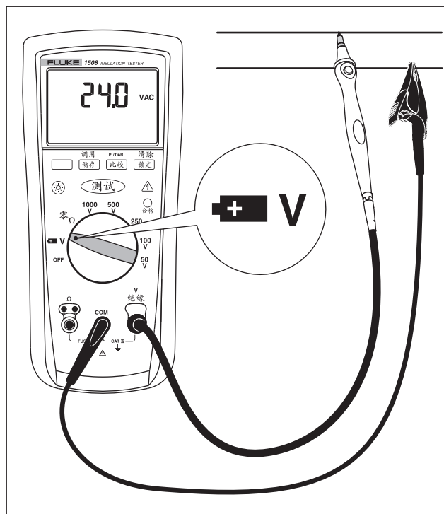
图 5. 测量电压
