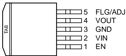
TO-263-5 (U)
