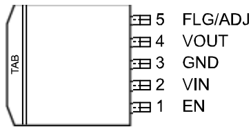
S-PAK-5 (R)
