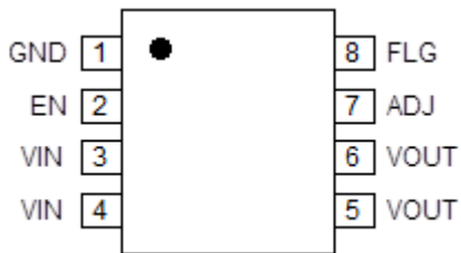
3mm x 3mm DFN (ML)
