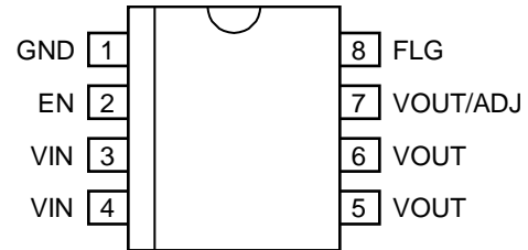
e-Pad SOIC-8 (ME)
