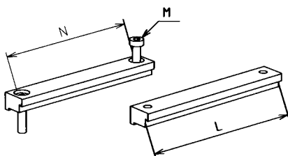
Ausführung mit Senkung version with counterbores
