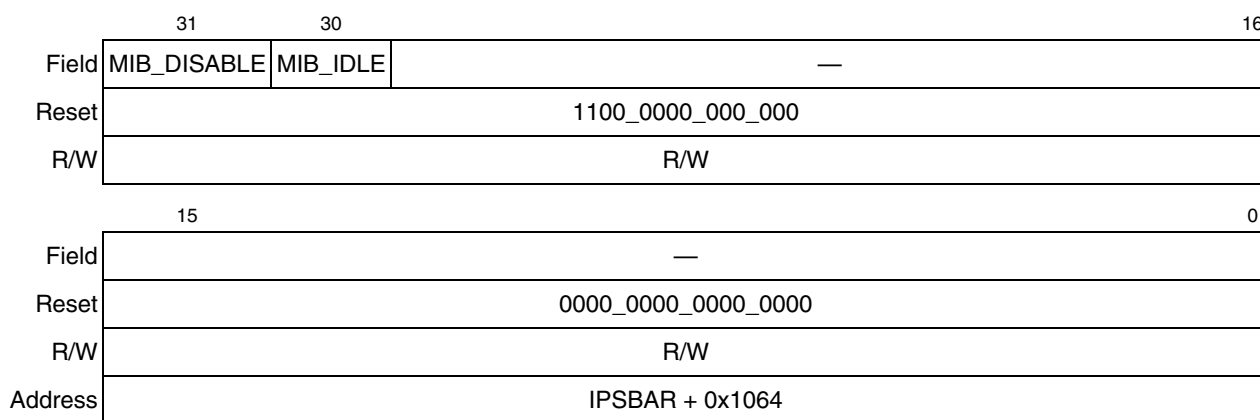
Figure 17-11. MIB Control Register (MIBC)
