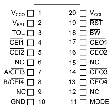
DS1321E 20-Pin TSSOP
