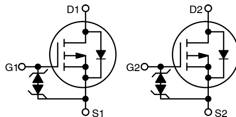
P-Channel MOSFET
