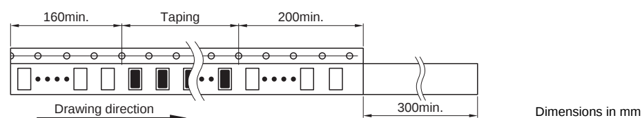
Type A B P1 K MMZ0603 0.38±0.05 0.68±0.05 2.0±0.05 0.5max.
