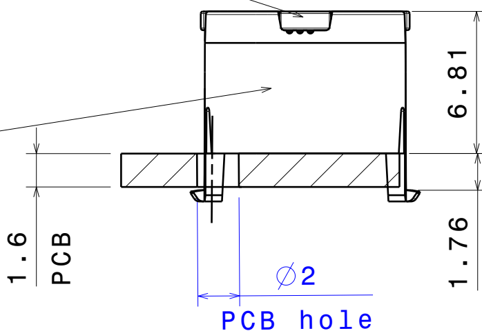
Front view Scale: 4:1
