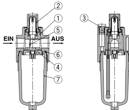
AL20
