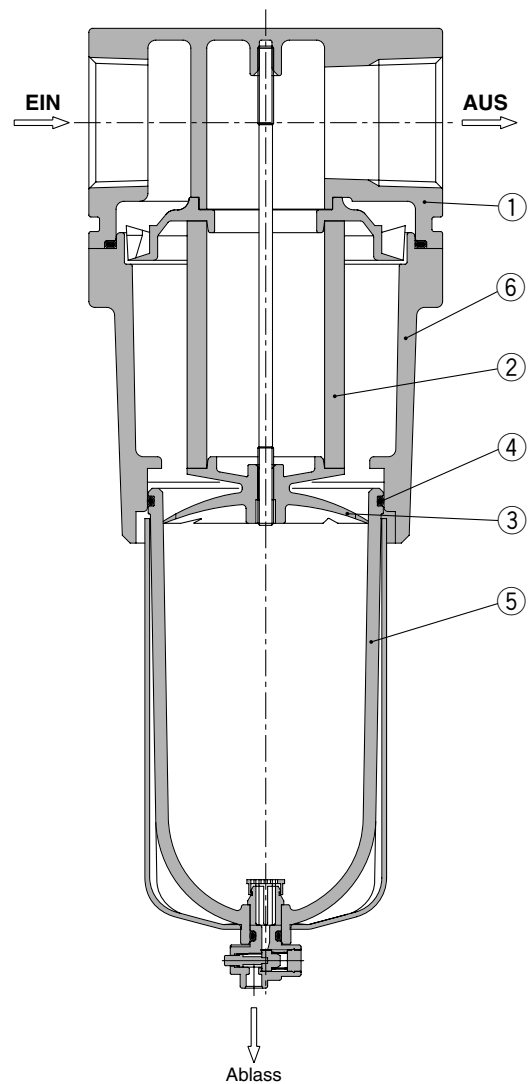
AF50, AF60
