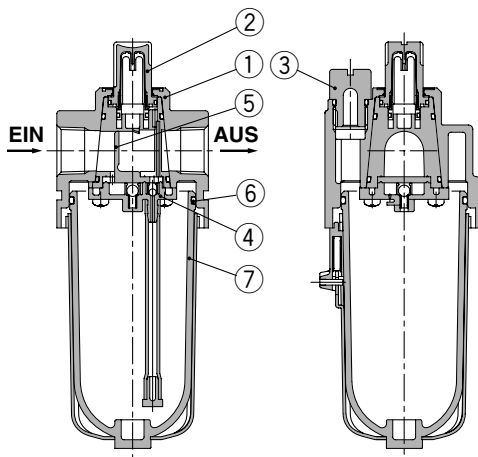
AL30, AL40
