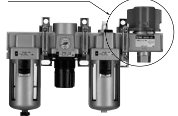
3/2-Wege Handabsperrventil
