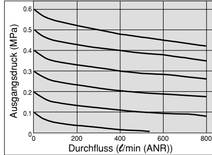
AC40 Rc 1/2
