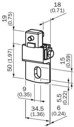
尺寸图 (尺寸单位: mm)
