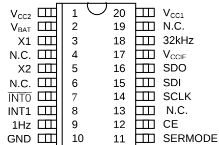
TSSOP (4.4mm)
