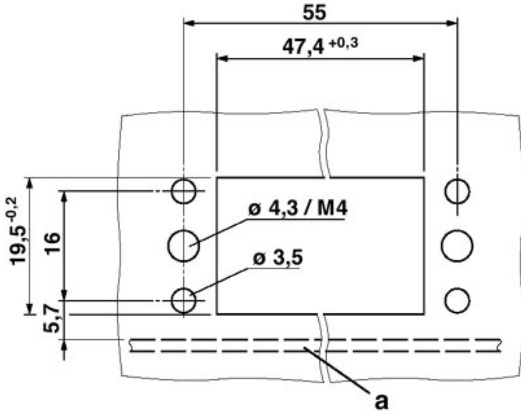
a - PCB
