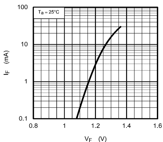
Fig. 13.1.3 I_F - V_F
