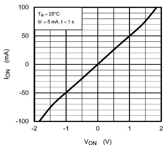
Fig. 13.1.4 I_{ON} - V_{ON}
