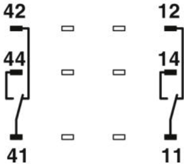
电路图
