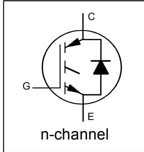
IRG8P60N120KDPbF TO-247AC
