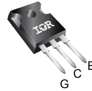
IRG8P60N120KDPbF TO-247AC
