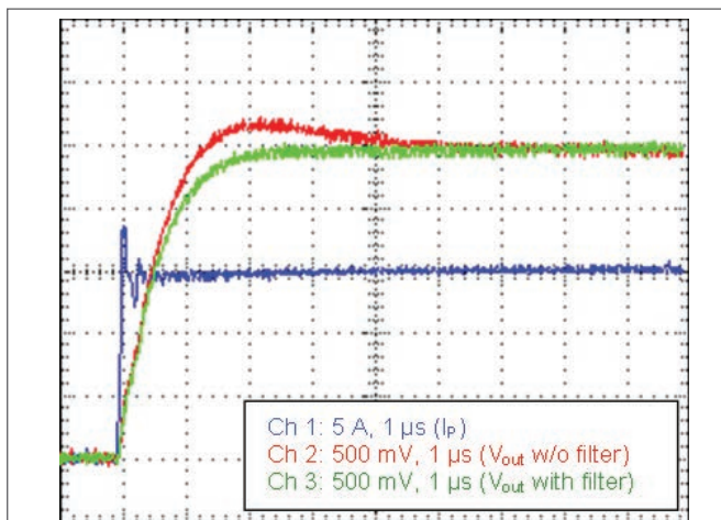
Fig. 4: Step response ( I_p = 15\text{ A} ; di/dt \sim 200\text{ A}/\mu\text{s} ; filter configuration acc. to Tab. 1).
