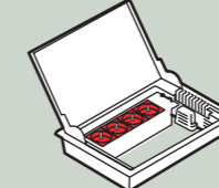
③ Montage dans la boîte
