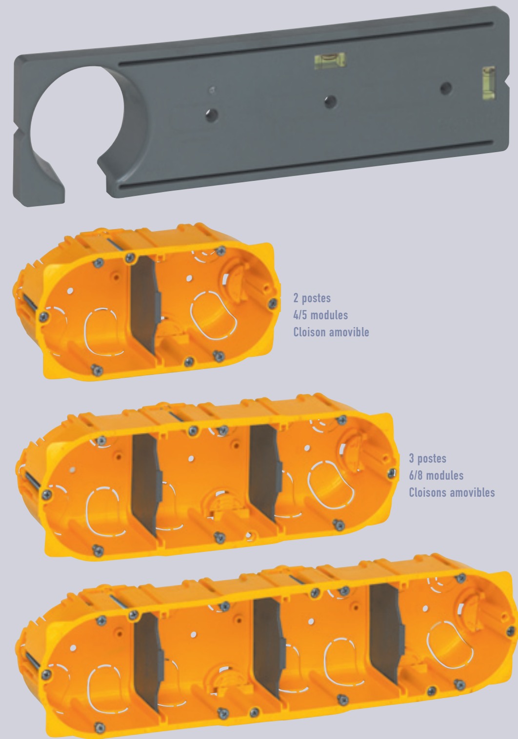
Gabarit facilitant la mise en œuvre des boîtes multipostes
