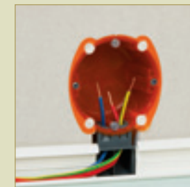
Mise en place de la moulure et des fils
