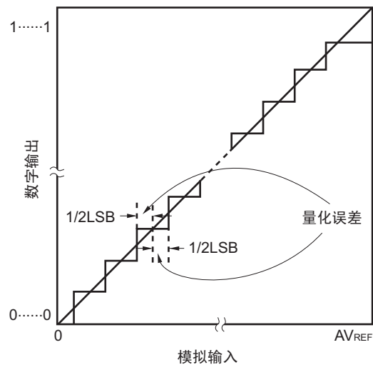
图 10-16 量化误差
