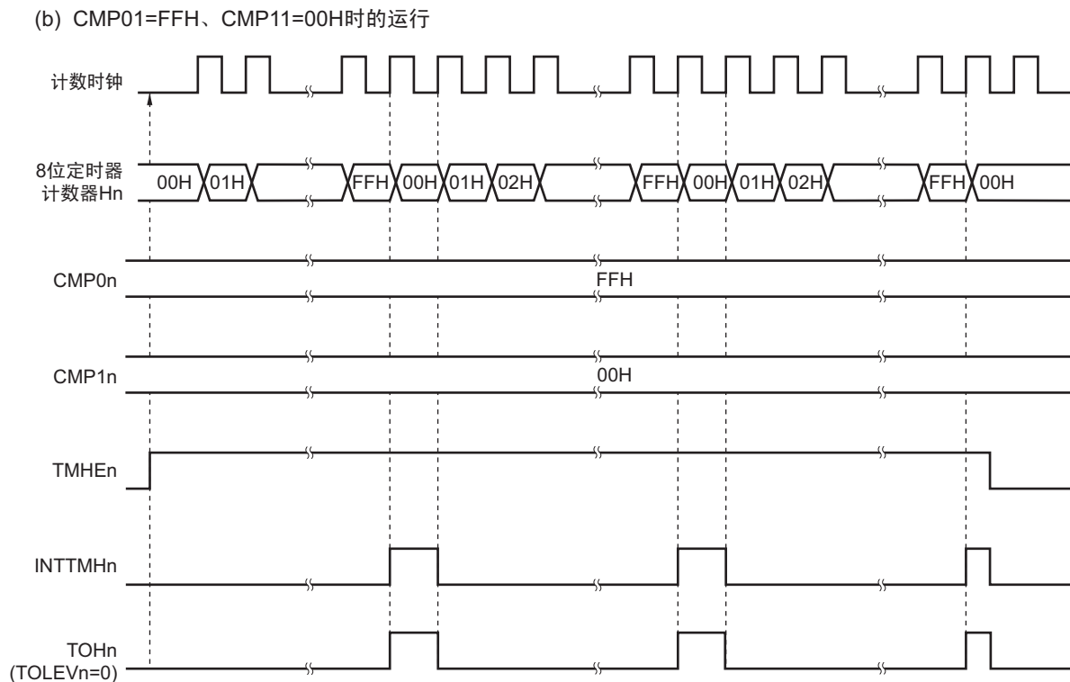
图 8-10 PWM 输出运行的时序 (2/4)
