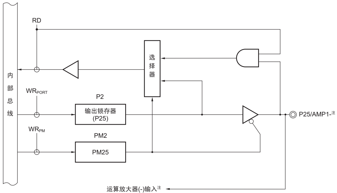
图 4-8 P25 的框图
