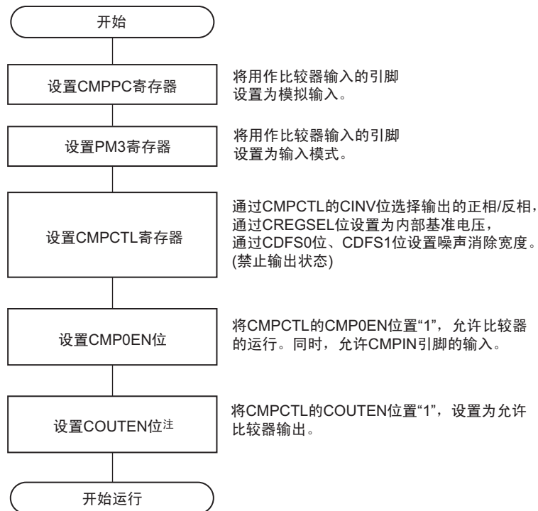
图 12-5 开始比较器运行的步骤示例（内部基准电压用作基准电压的情况）
