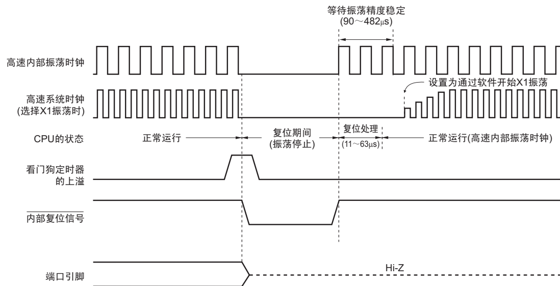
图 16-3 通过看门狗定时器上溢进行的时序
