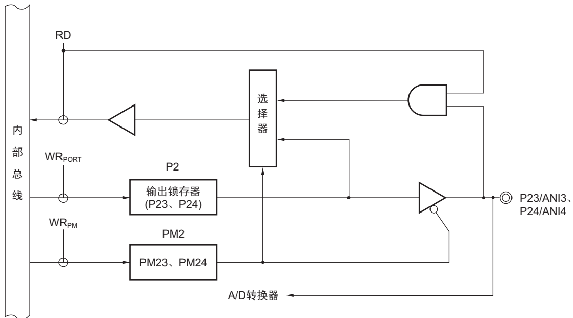
图 4-7 P23、P24 的框图
