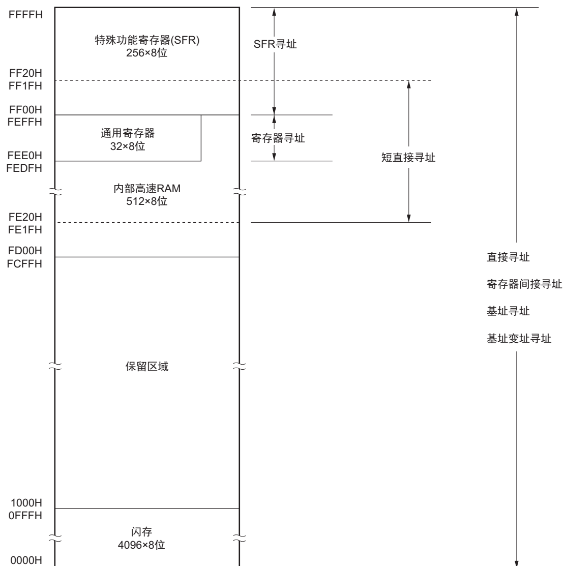
图 3-4 数据存储与寻址的对应（R7F0C300x、R7F0C303x、R7F0C306x、R7F0C309x）
