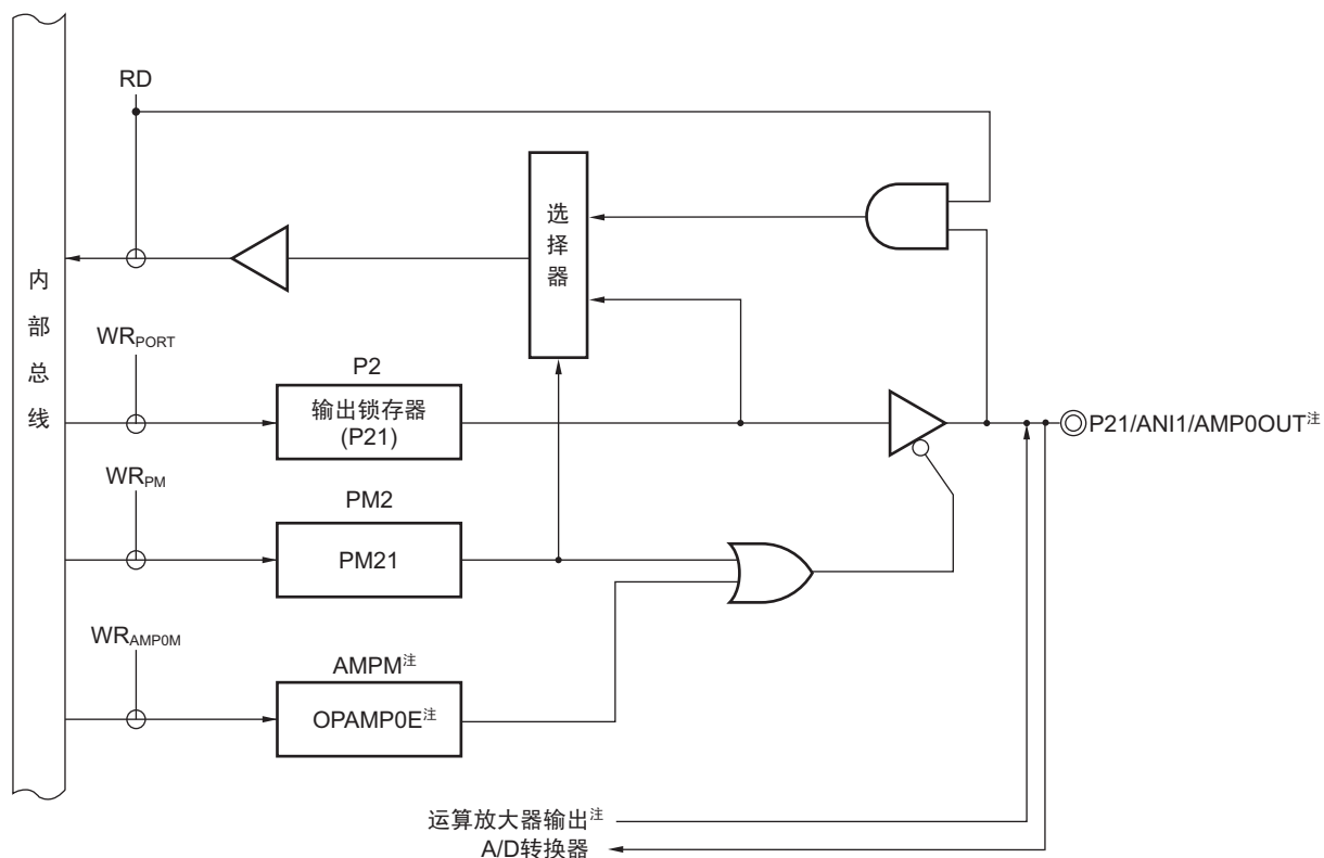
图 4-5 P21 的框图
