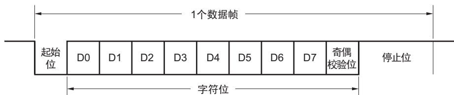
图 13-6 正常 UART 发送 / 接收数据的格式
