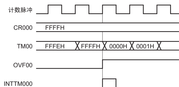
图 6-58 OVF00 标志的变化时序
