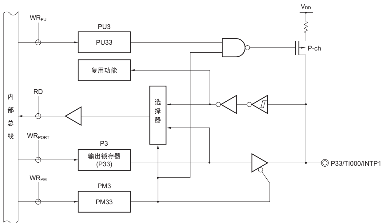
图 4-14 P33 的框图
