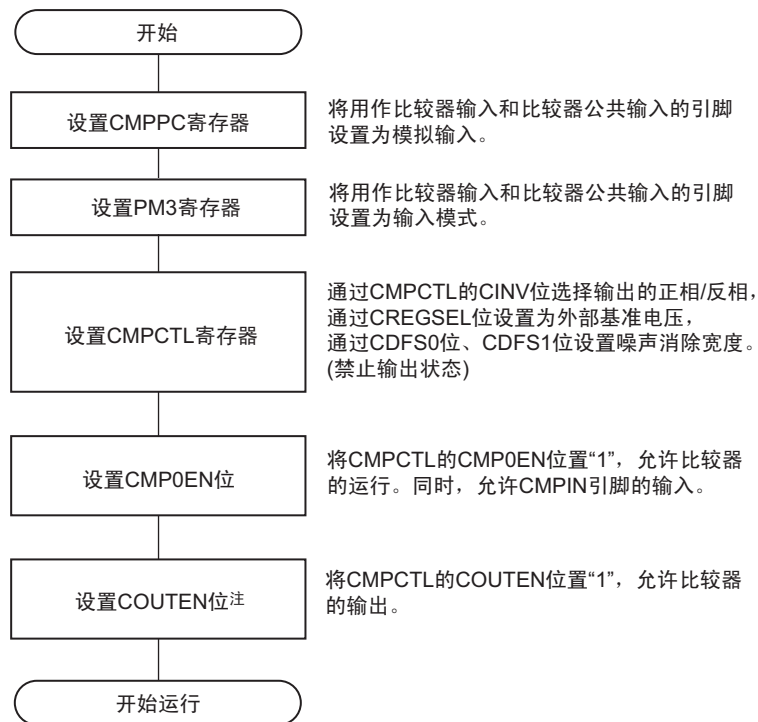
图 12-6 开始比较器运行的步骤示例 （比较器公共引脚（CMPCOM）的输入电压用作基准电压的情况）
