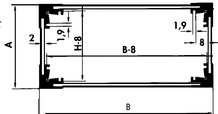
Eckprofil / Edge Profile / Profile d'angle G 1 B
