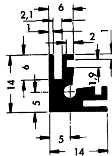
Eckprofil / Edge Profile / Profile d'angle G 1 B
