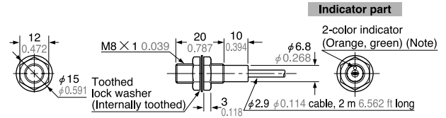
GX-8MU GX-8MUB Sensor
