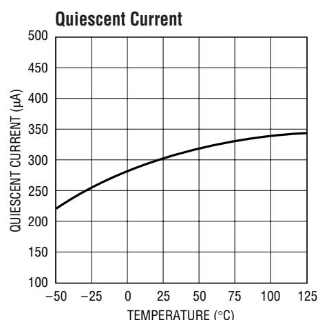
LT1111 • TPC11
