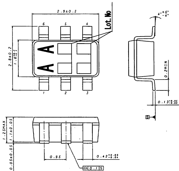
SSOP6 (UNIT:mm)
