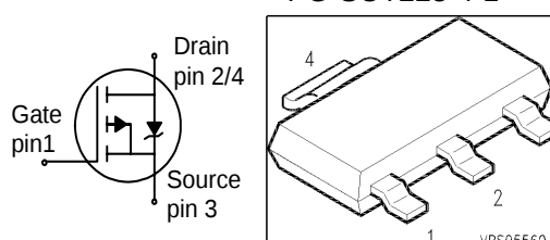
PG-SOT223-4-1
