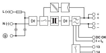
结构框图
