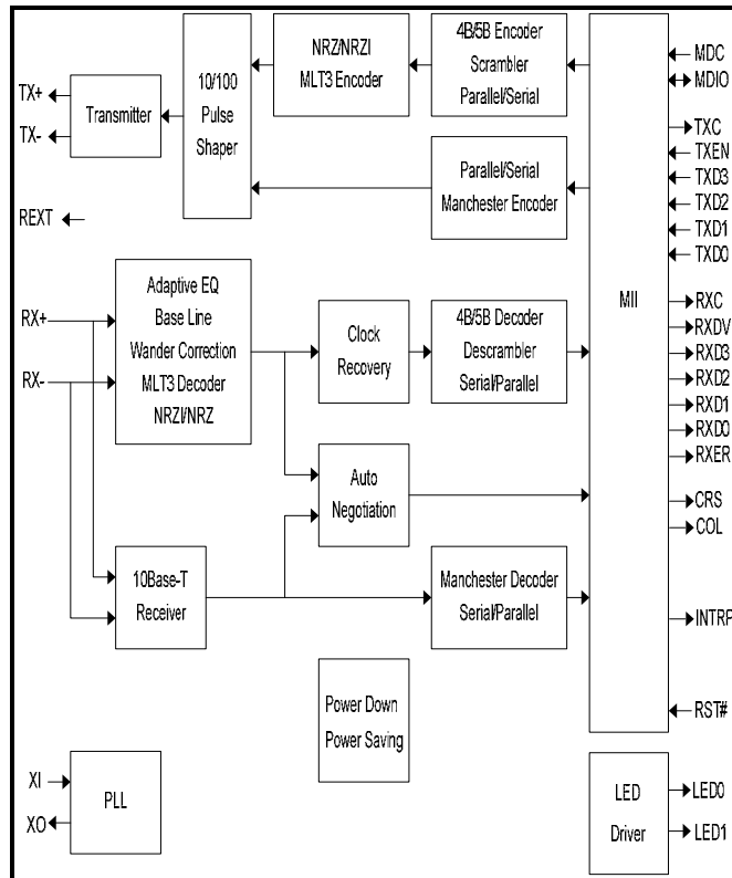
KSZ8041MLL
