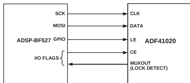
Figure 19. ADSP-BF527-to-ADF41020 Interface
