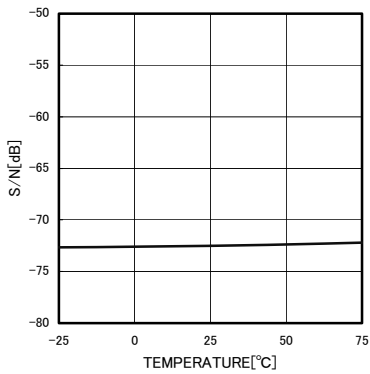
Fig.18 S/N
