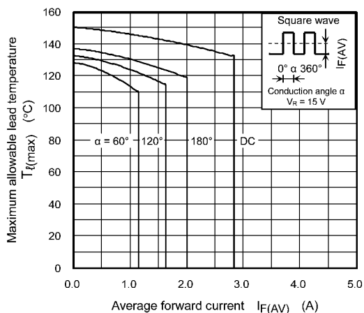
Fig. 10.4 T_{t(max)} - I_{F(AV)}
