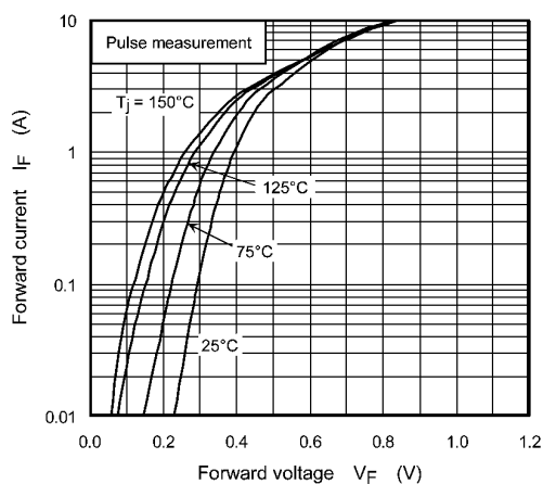
Fig. 10.1 I_F - V_F
