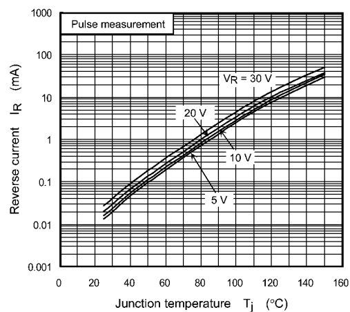
Fig. 10.8 I_R - T_j
