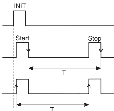
Bild 2-1: Zeit-/Wegmessprinzip
