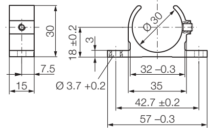
Bild 8-2: Befestigungsklammer BTL6-A-MF01-A-43
