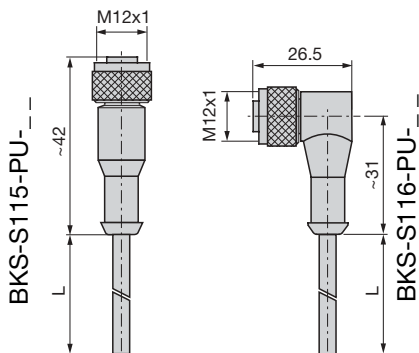
Bild 4-2: Anschlusskabel BKS-S...
