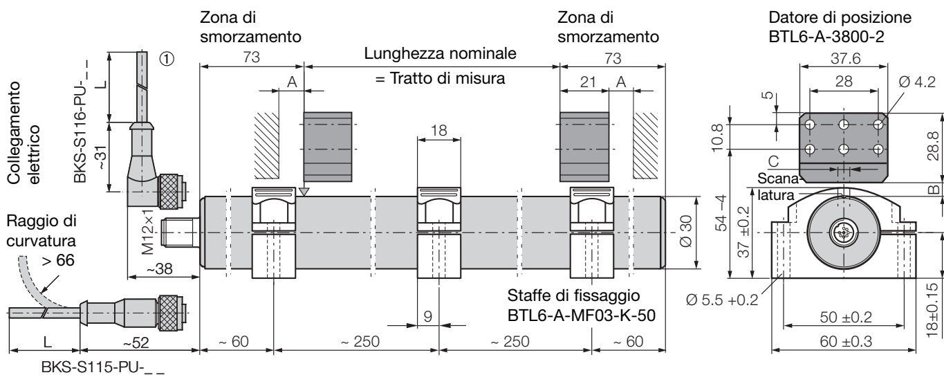
Fig. 3-1: Disegno quotato (trasduttore di posizione BTL6...A1-S115 con datore di posizione BTL6-A-3800-2 e staffe di fissaggio BTL6-A-MF03-K-50)
