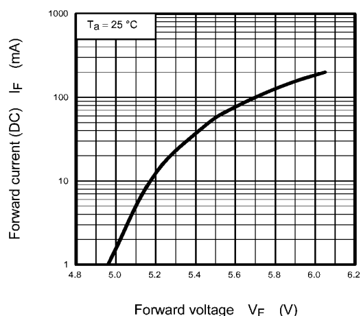
Fig. 8.1 I_F - V_F
