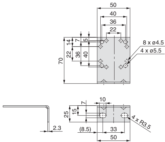
L-bracket
