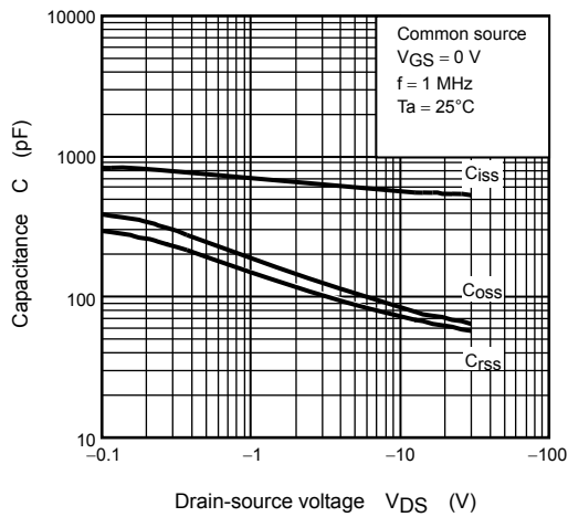
Capacitance - V_{DS}
