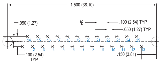
25 SOCKET M83513/25-D
